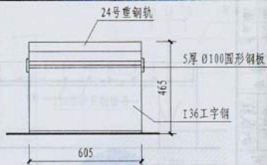
侧立面图
