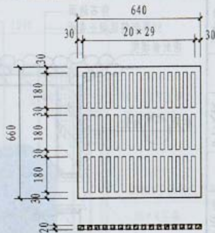
Ⓐ 铸铁算子
