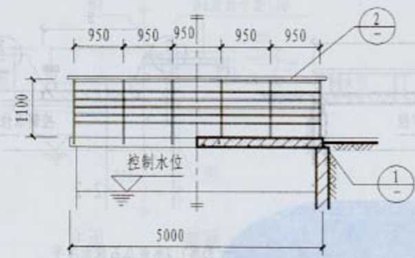
立面 1-1
