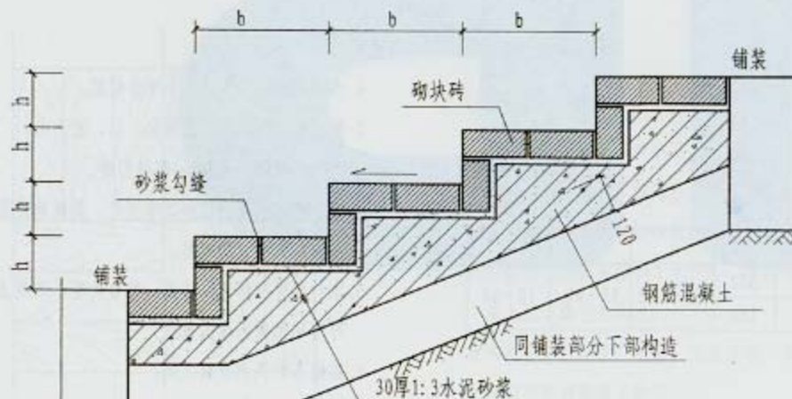
① 混凝土台阶
