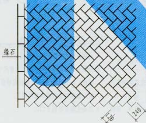
④ 卧铺
