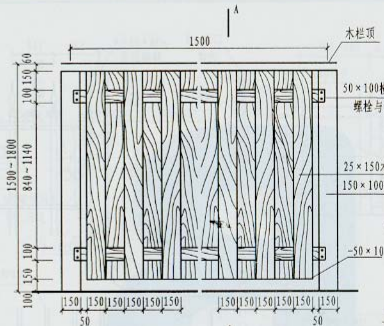
② 立面
