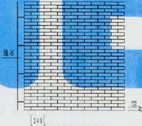
⑤ 立铺
