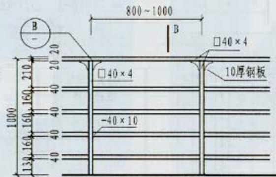
6 立面
