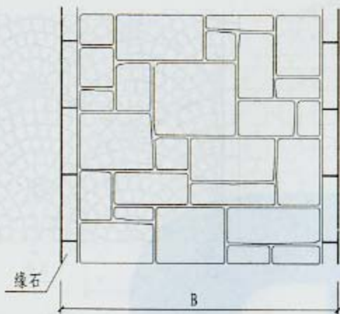
① 料石
