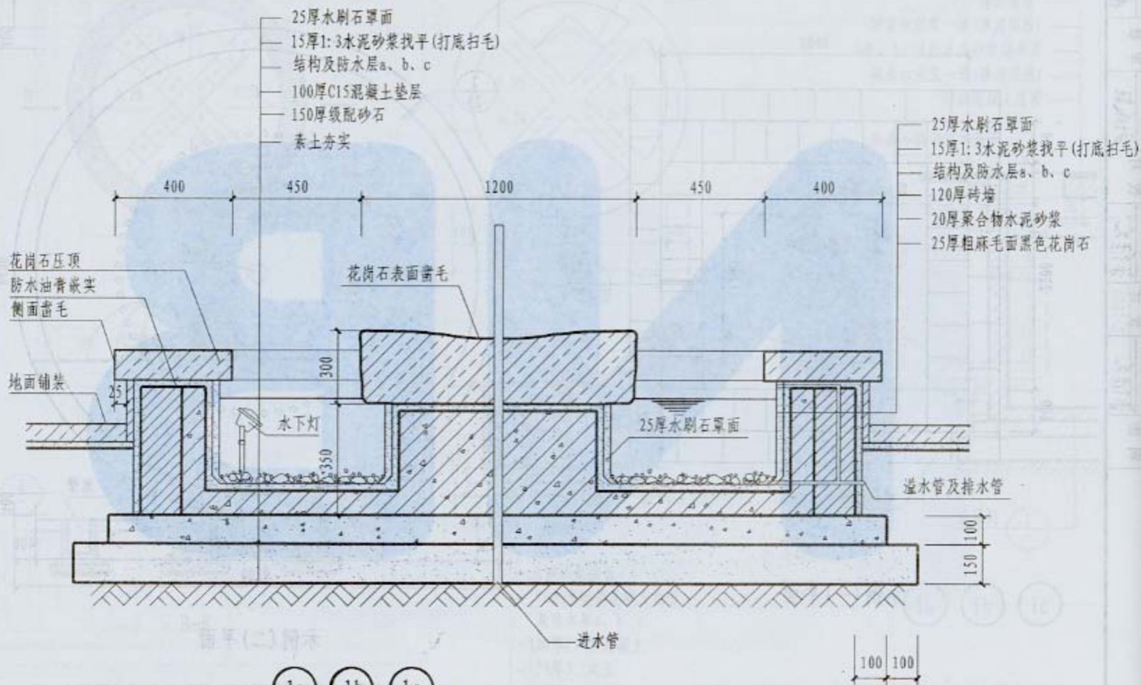
喷泉示例(一)剖面图
