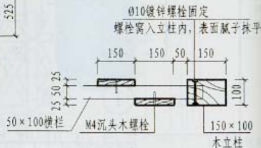
④ 节点详图
