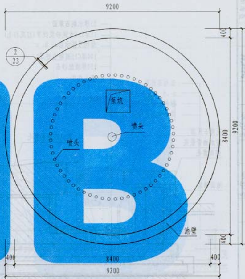
示例(二)平面
