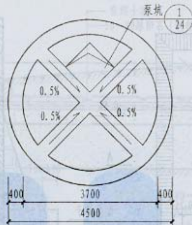
坑底平面
